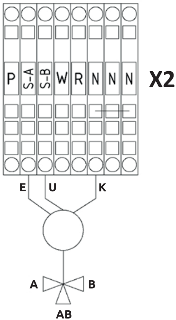
Малюнок 24 – Електропідключення приводу триходового клапана.
