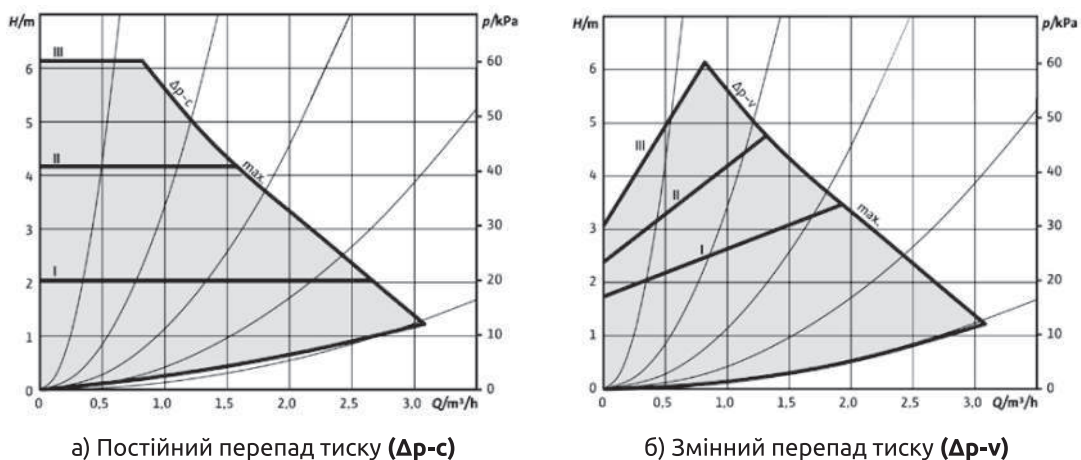
Малюнок 9 – Характеристика насоса Wilo PARA 15-130/6-43/SC для режимів.
