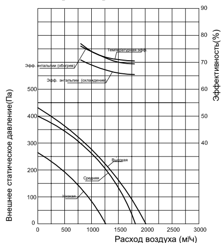
CH-HRV15K2 (CH-HRV15AK2) Диаграмма производительности
