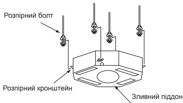
Рис. 3.8. Монтаж внутрішнього блоку
