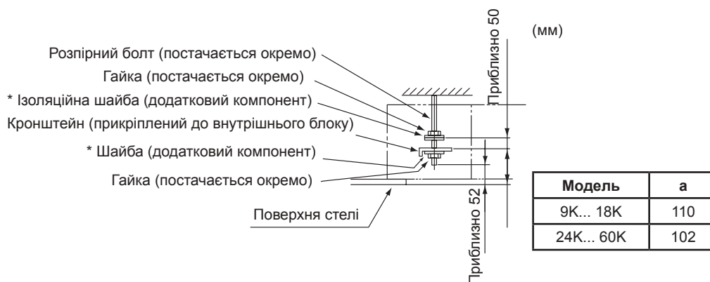
Рис. 3.7. Монтаж гайок і шайб
