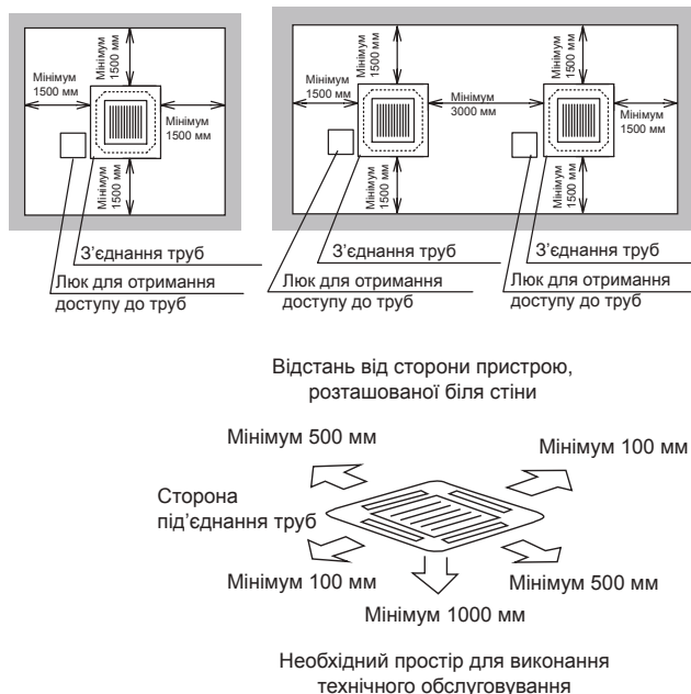
Рис. 3.1. Простір навколо внутрішнього блоку
