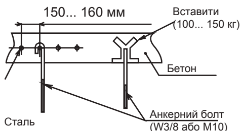
Рис. 3.4. Встановлення розпірних болтів
