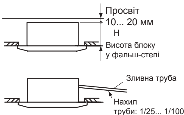
Рис. 3.2. Місце встановлення внутрішнього блоку
