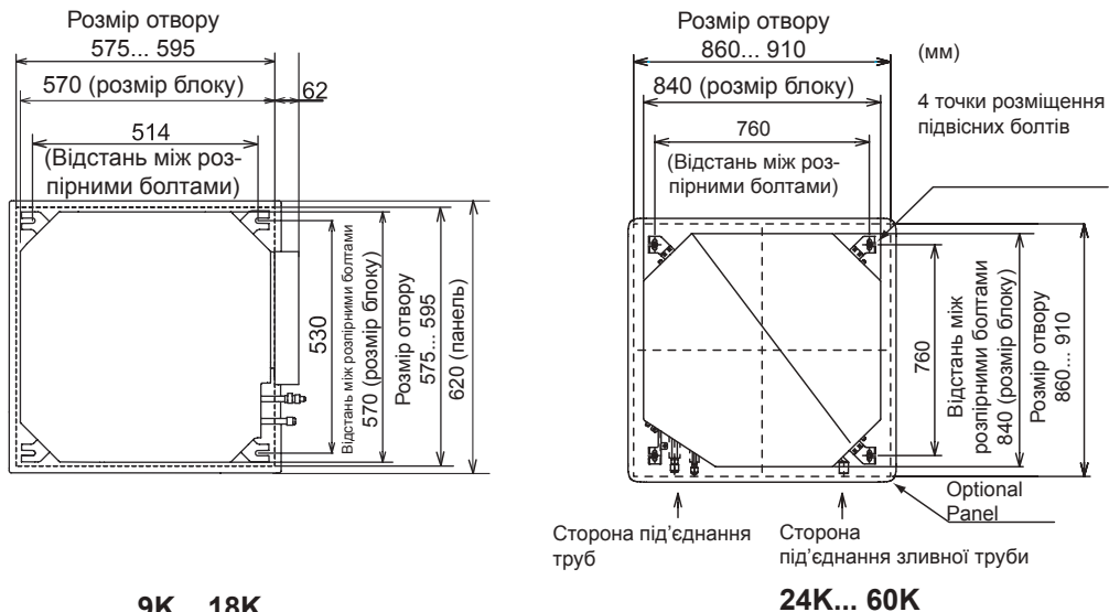
Рис. 3.3. Підготовка отвору у фальш-стелі та монтаж розпірних болтів
