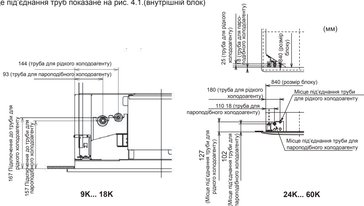
Рис. 4.1 Місце під'єднання труб
