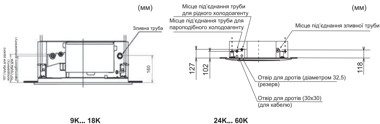
Рис. 3.6. Внутрішній блок і вентиляційна решітка
