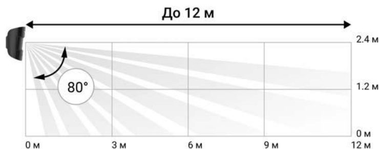
Вертикальний кут огляду датчика
