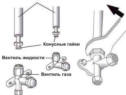
Соединительные трубы
