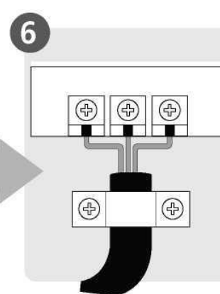
Під'єднання кабелю
