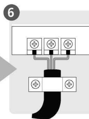
Під'єднання кабелю
