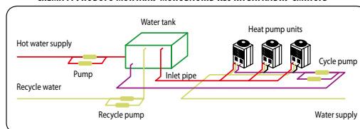
СХЕМА ГРУПОВОГО МОНТАЖУ МОНОБЛОКІВ RSJ НА ЗАГАЛЬНУ ЄМНІСТЬ
