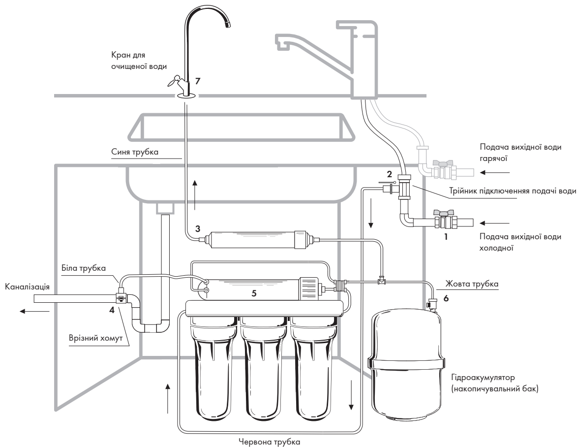
Рис. 2. Загальний вигляд підключеної системи Organic Master Osmo 5
