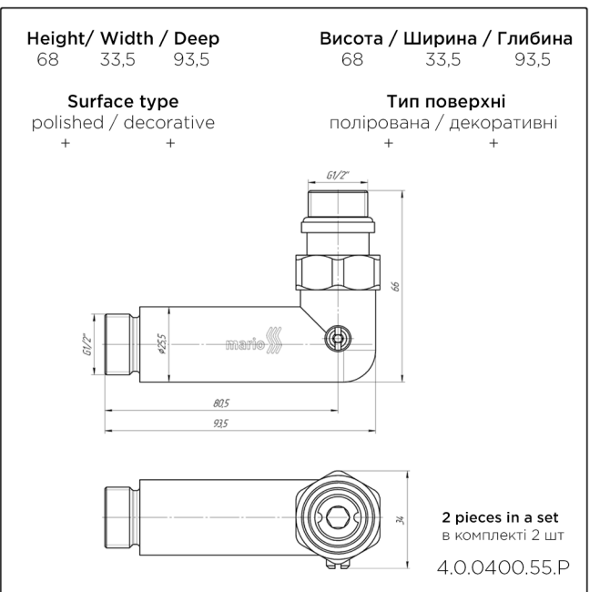
Shut-off angled valves set Комплект кранів кутових запірних
