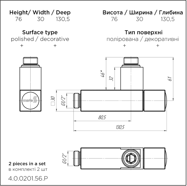
Square angled valves set Комплект кранів регулюючих кутових квадратних
