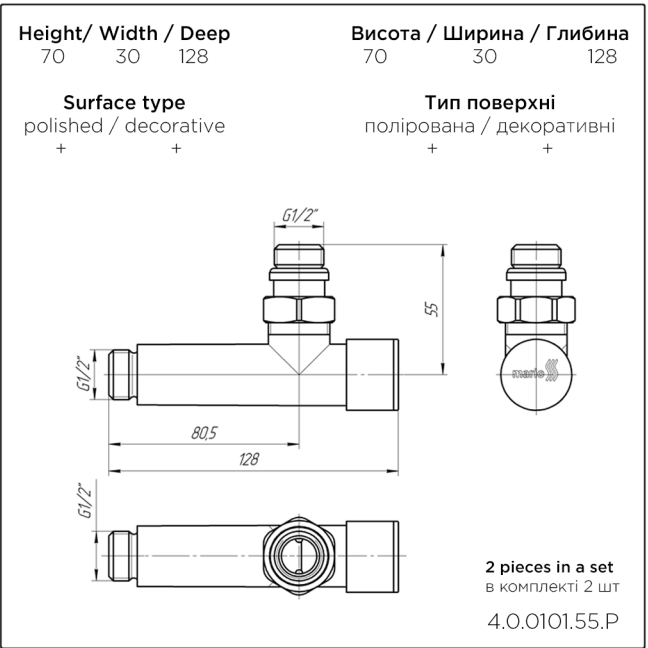
Round angled valves set Комплект кранів регулюючих кутових круглих
