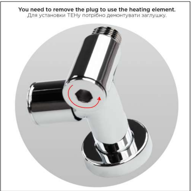
The heating element can be installed only into the pipe riser with a "heating element" sticker. Розташувати ТЕН можна лише в стояк, на якому є наліпка «ТЕН».
