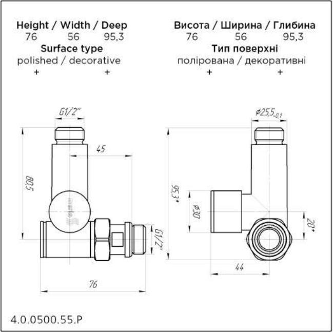
You need to remove the plug to use the heating element. Для установки ТЕНу потрібно демонтувати заглушку.
