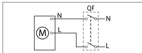
Альта 100... Т (ТН, Т1)
