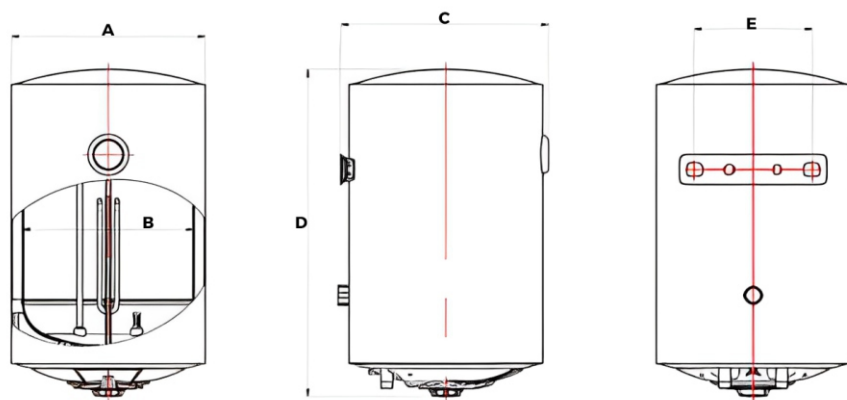
Рисунок 1. Габаритні розміри (Тип встановлення: вертикальний)
