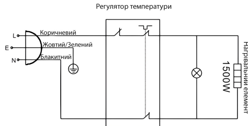
Рисунок 4. Схема підключення
